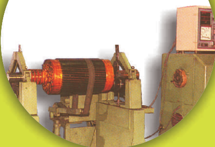
Balaceador eletrônico
